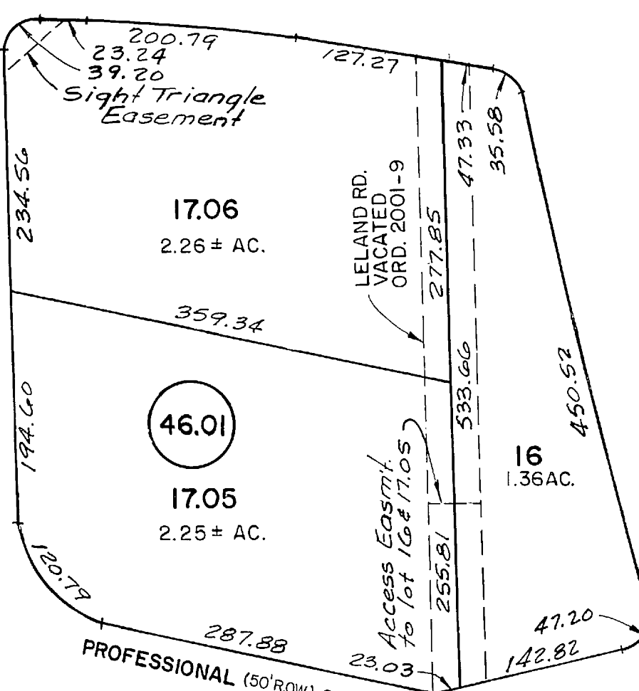
INSET "A" BLOCK 46.01 N.T.S.
