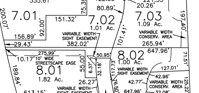
INSET "B" BLOCK 48 N.T.S.
