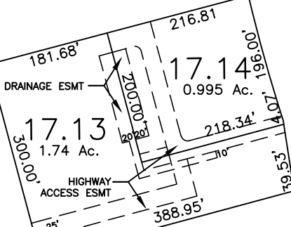
INSET "C" BLOCK 46 N.T.S.
